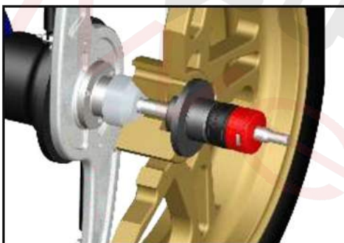
Wał ze specjalnym zestawem centrującym.
