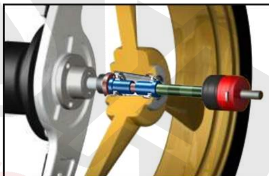
Wał z tulejami centrującymi.
