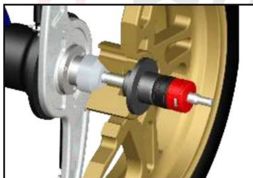
Wał ze specjalnym zestawem centrującym.
